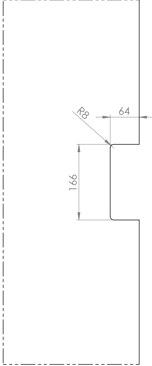
1540 CAM KESİDİ
