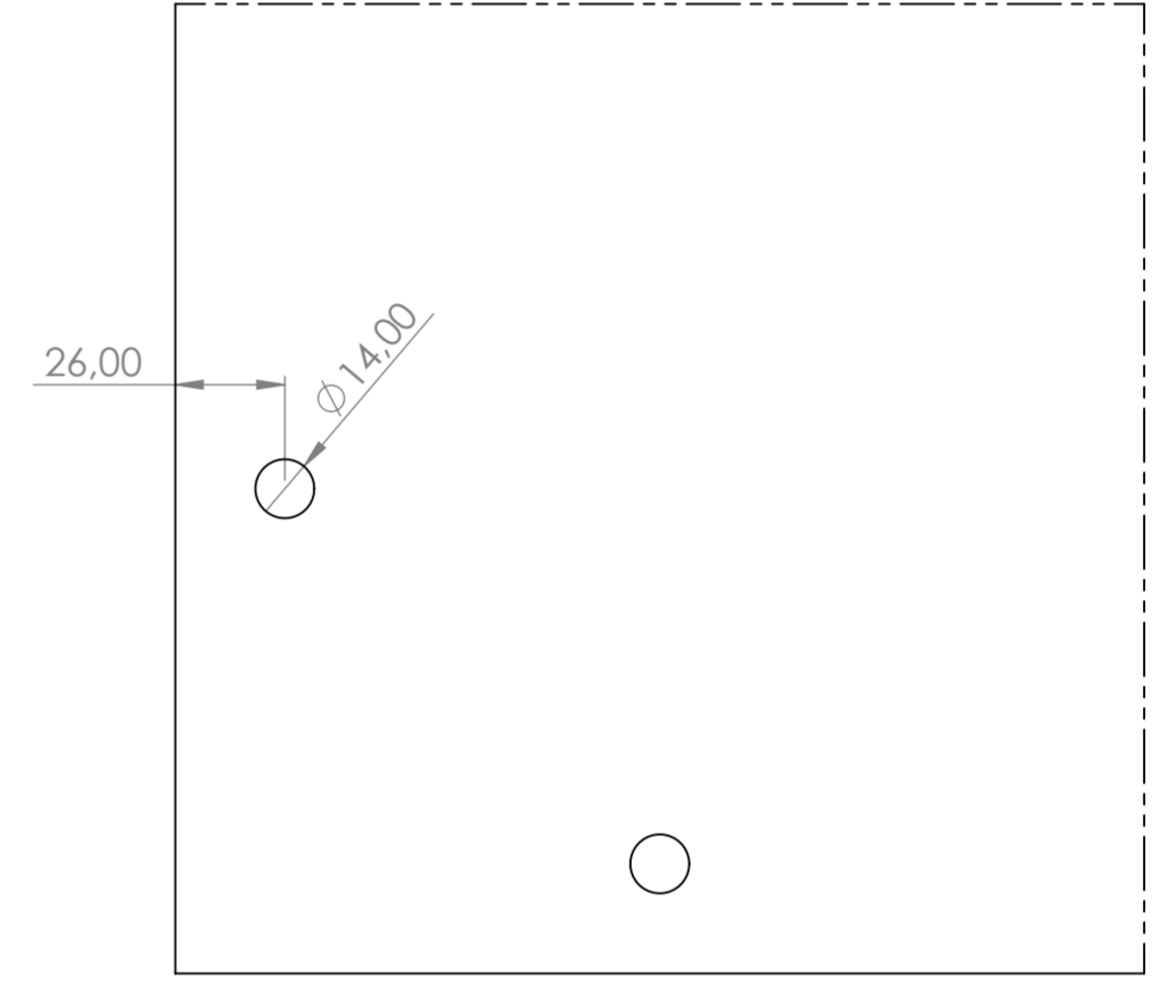
CAM KESİDİ
