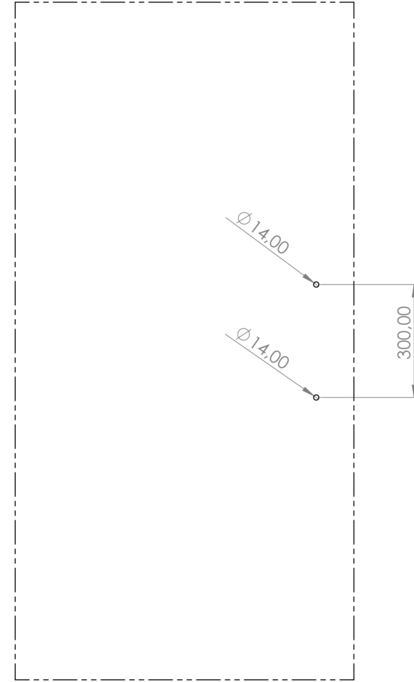
CAM KESİDİ
