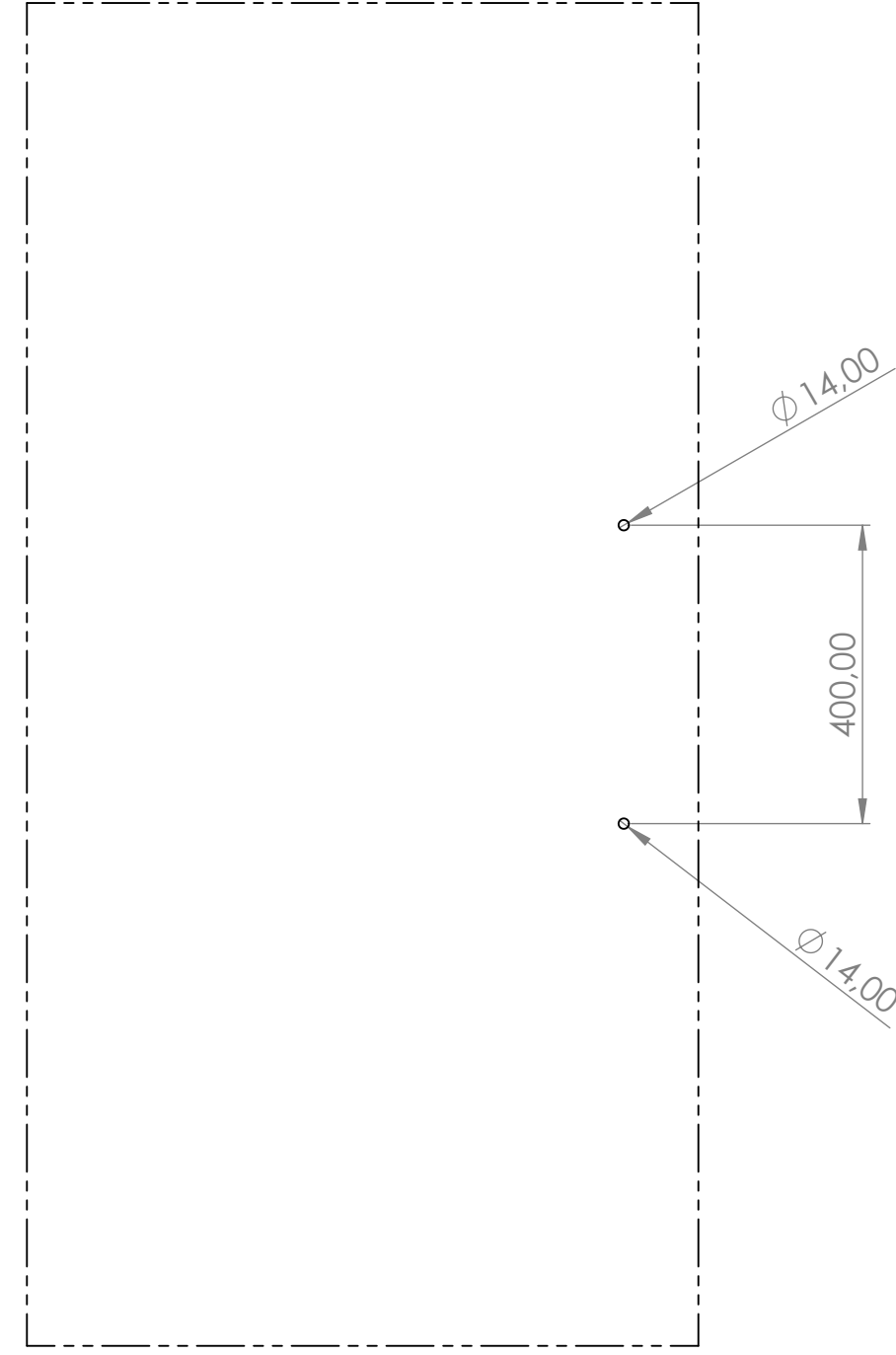
CAM KESİDİ
