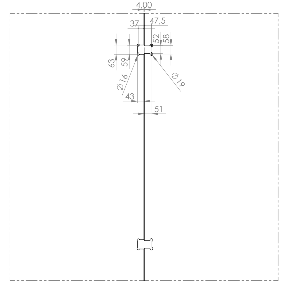
CAM KESİDİ
