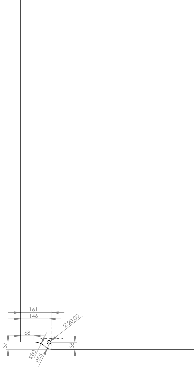
6200 CAM KESİDİ
